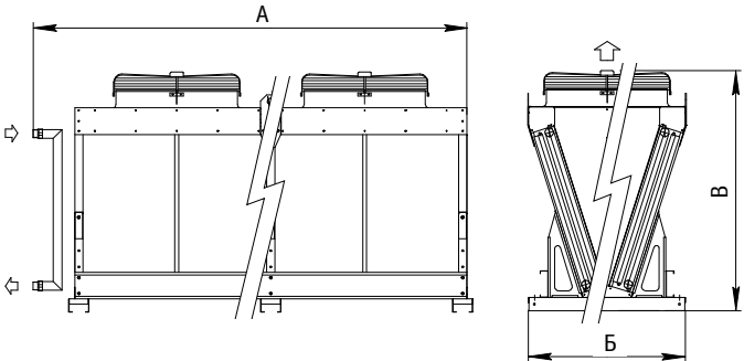
Драйкулеры V-образные
